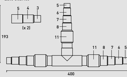
Lato scarico
