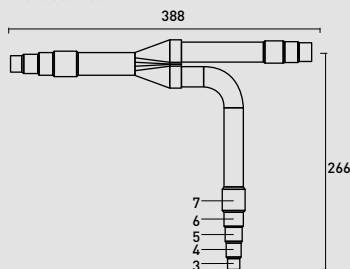
Lato scarico
