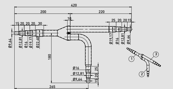
Lato liquido
