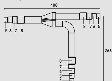
Lato aspirazione
