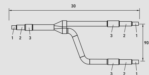
Lato liquido
