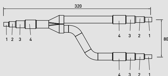
Lato liquido
