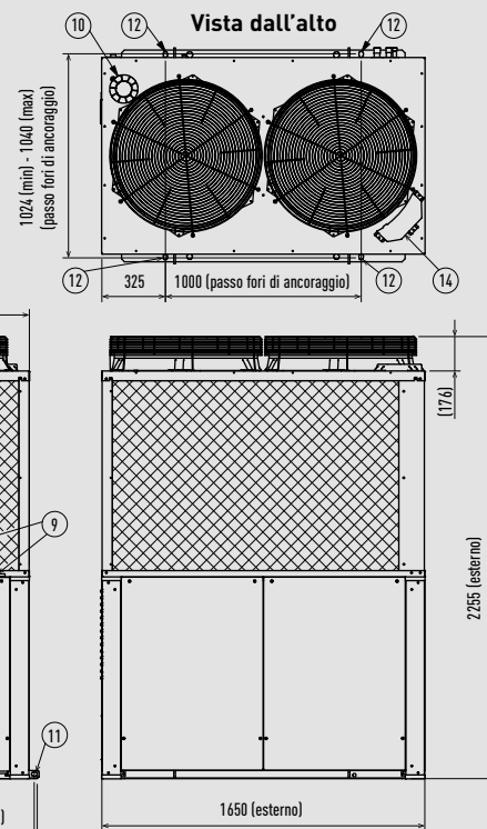
Vista frontale
