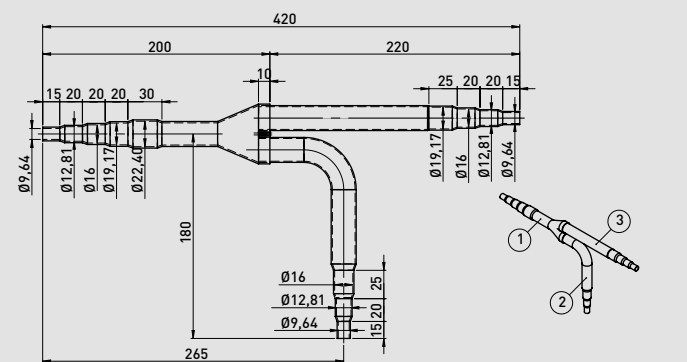
Lato liquido
