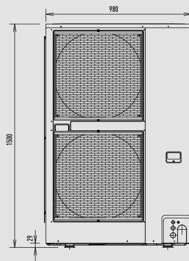
Vista frontale
